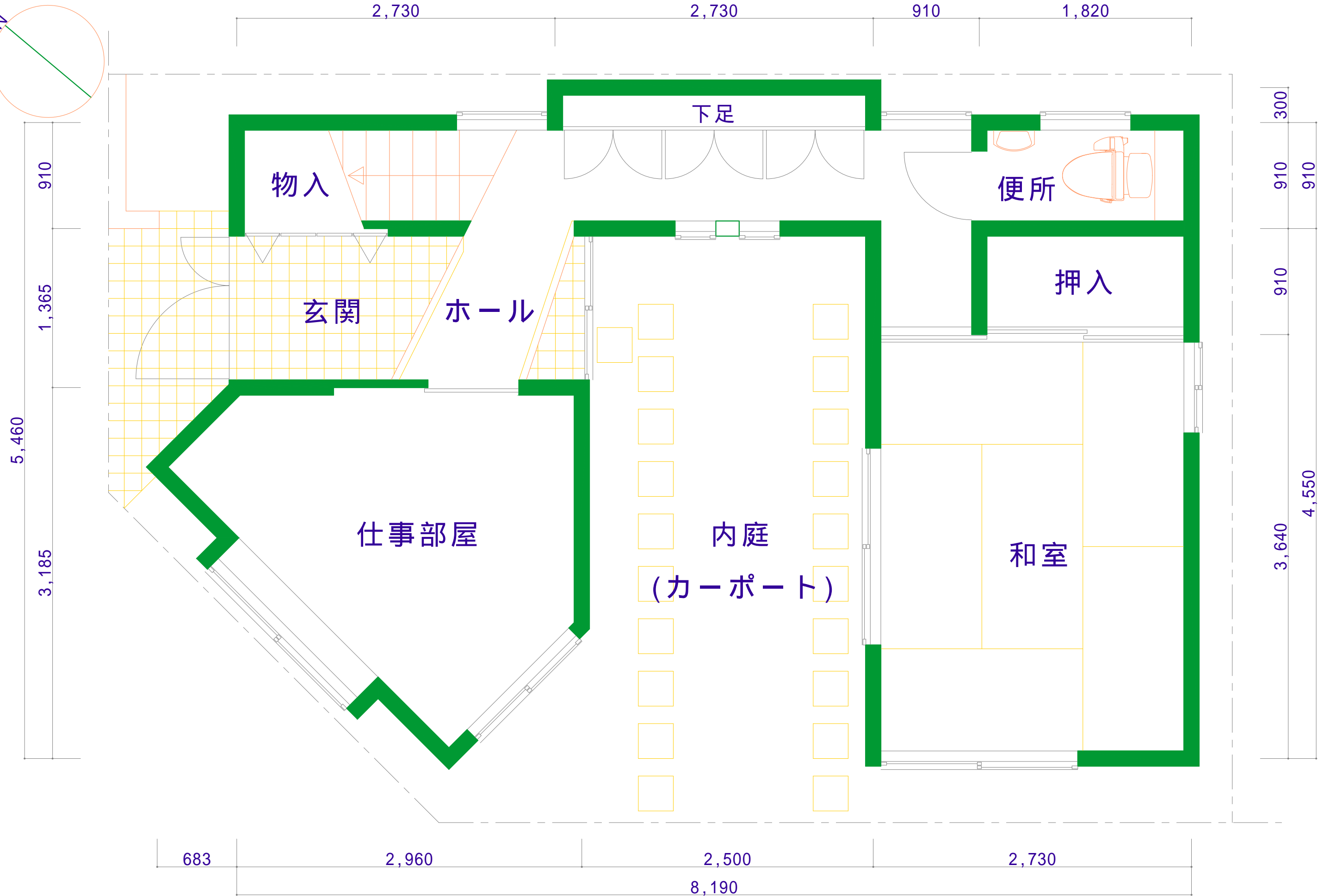
1階平面図
