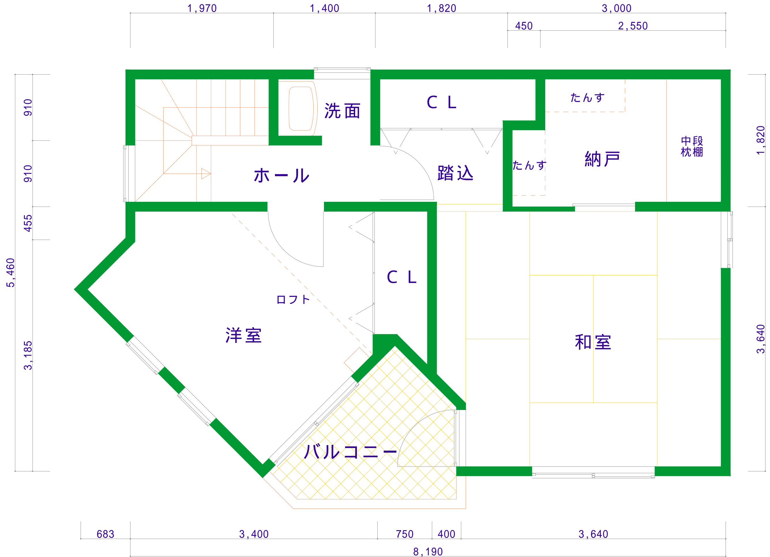
3階平面図
