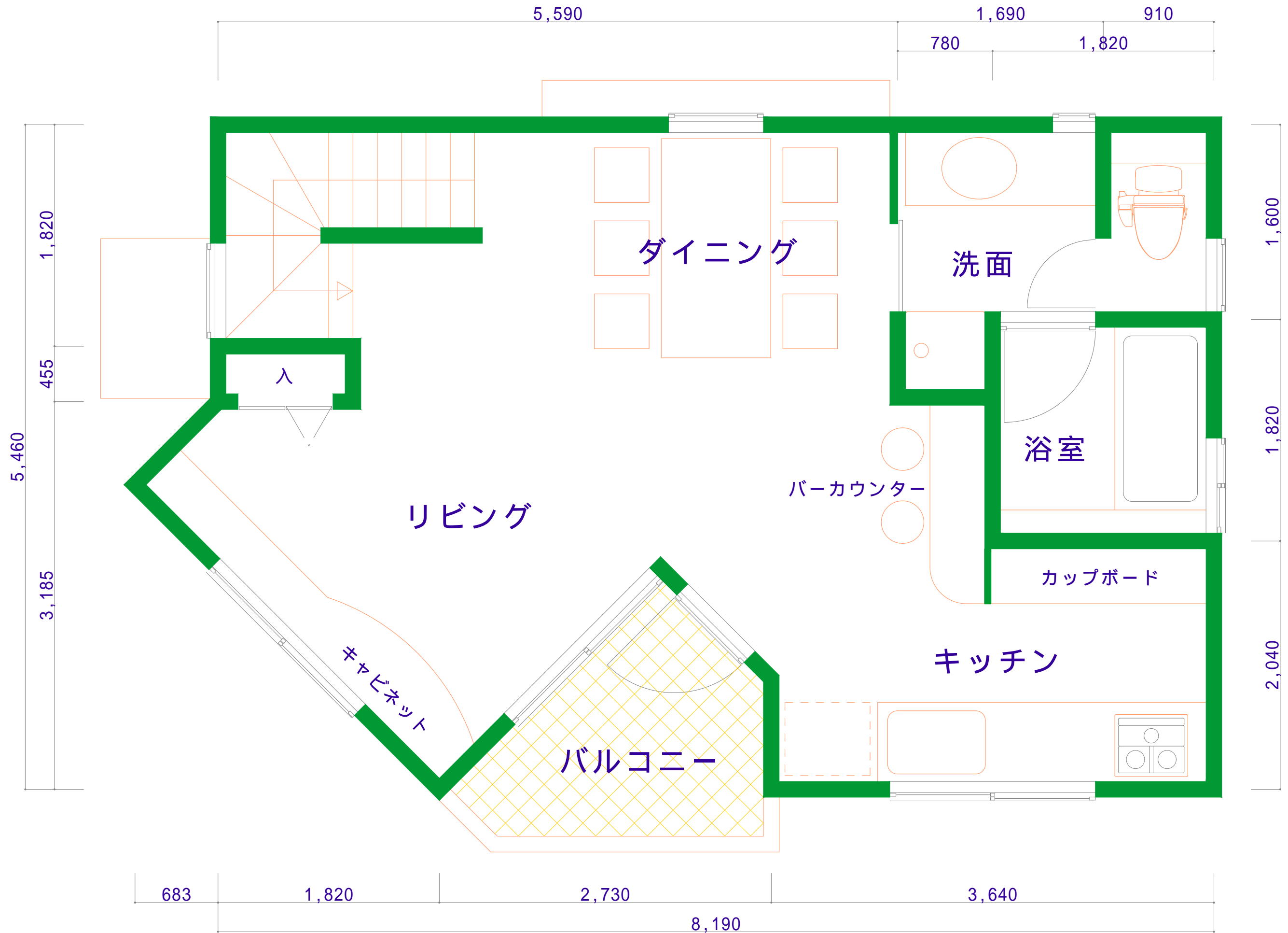
2階平面図
