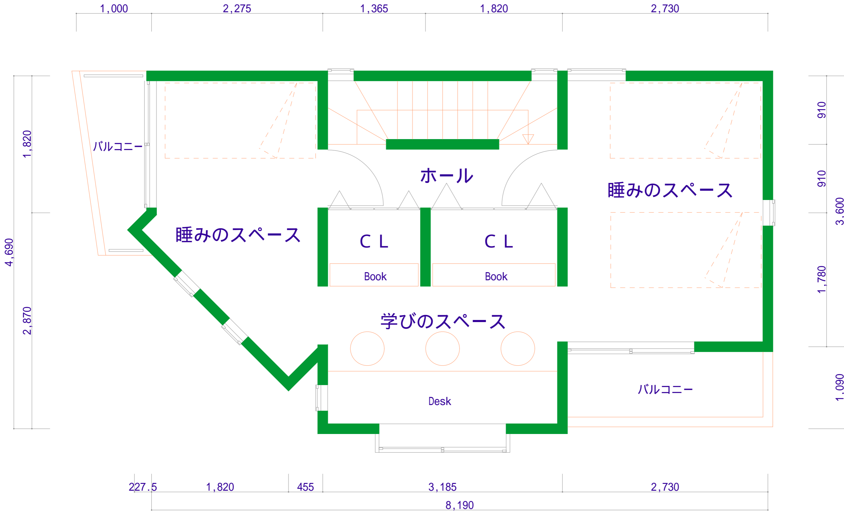
2階平面図
