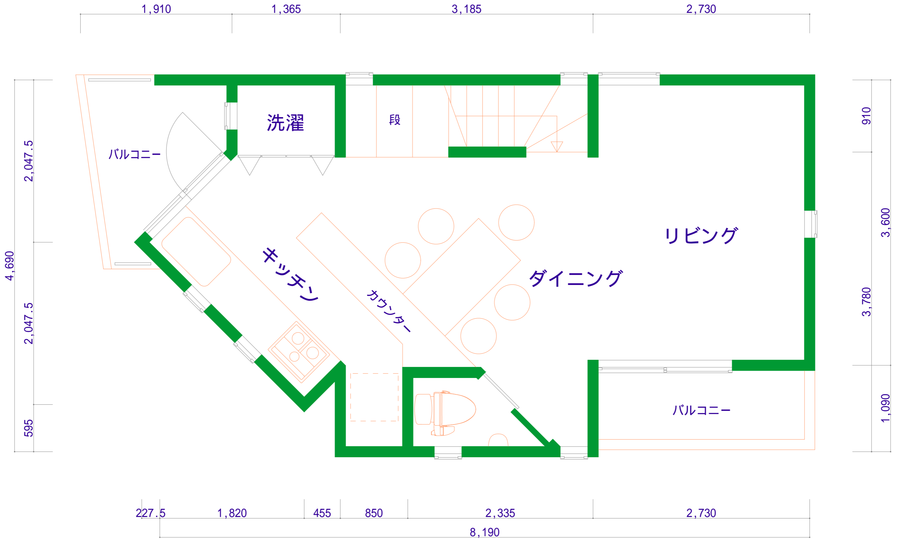
3階平面図
