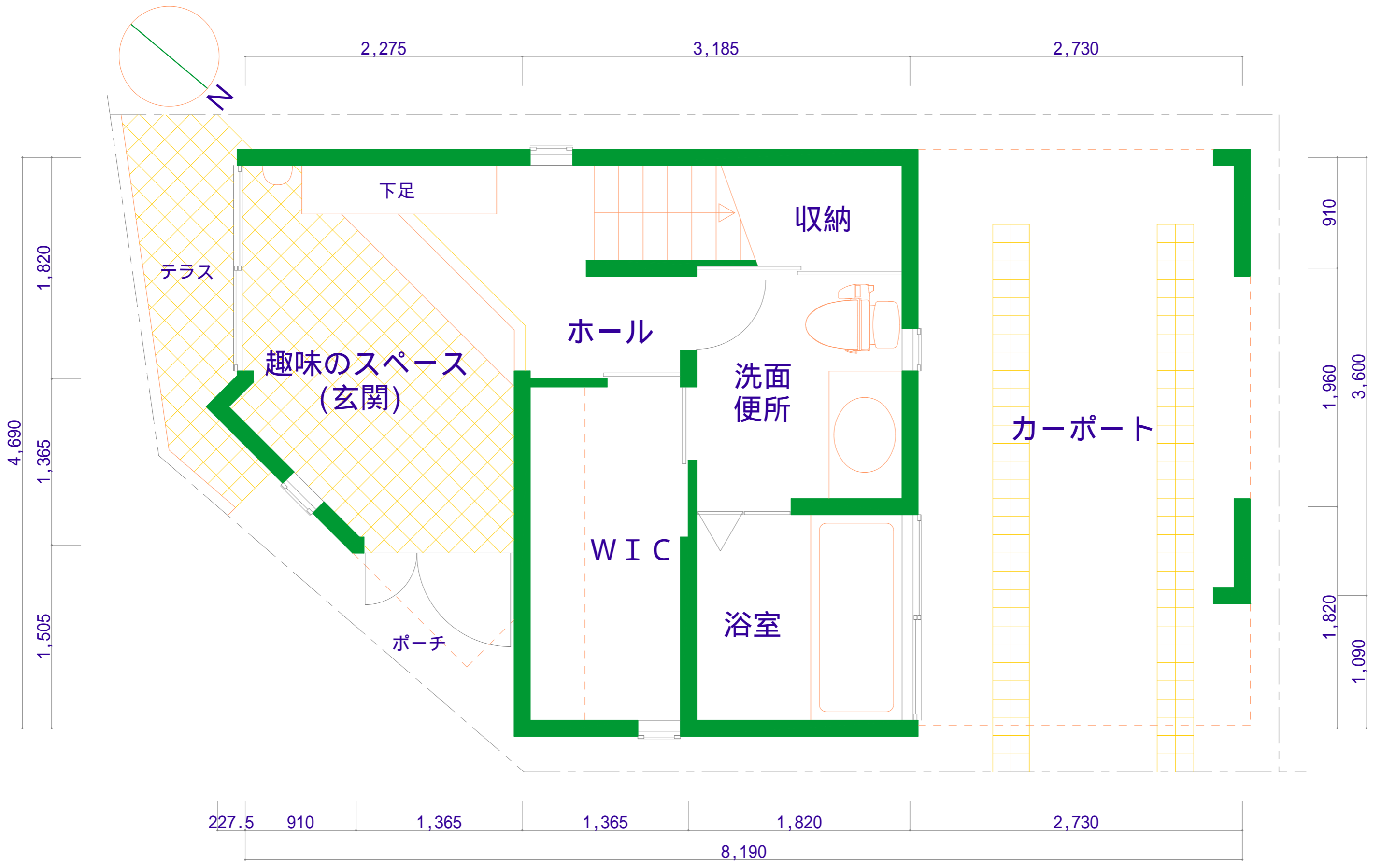
1 階平面図
