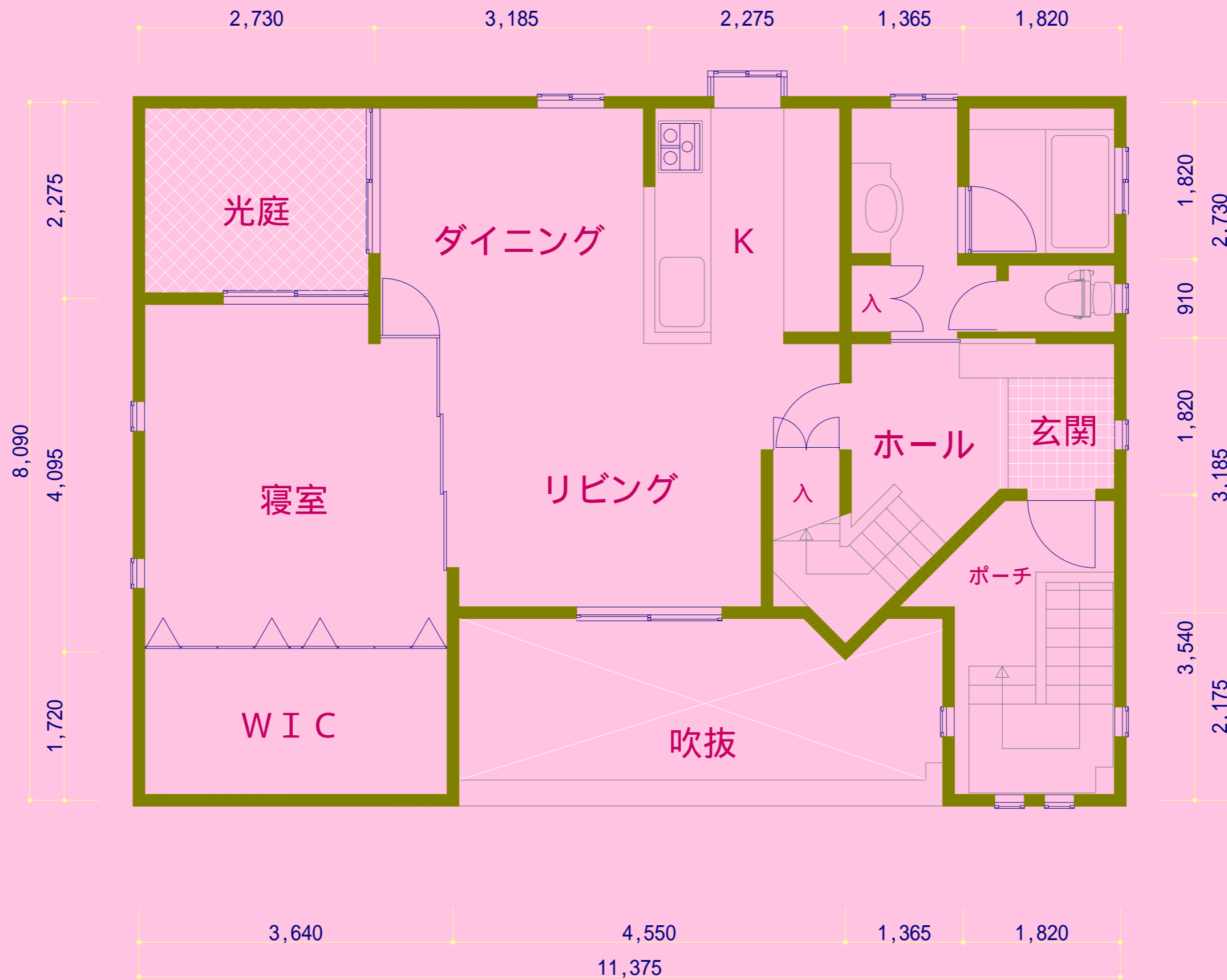
2階平面図
