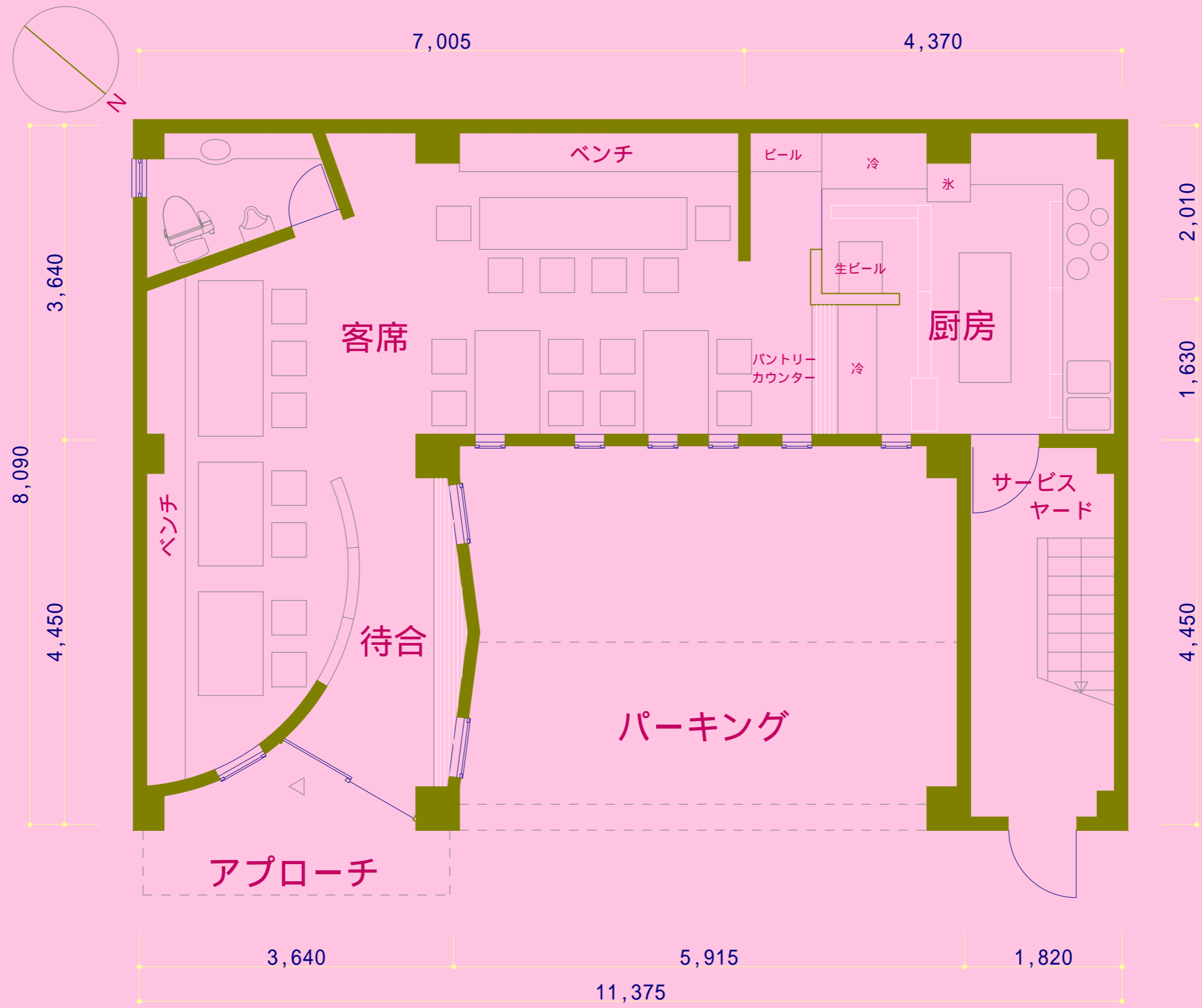
1階平面図
