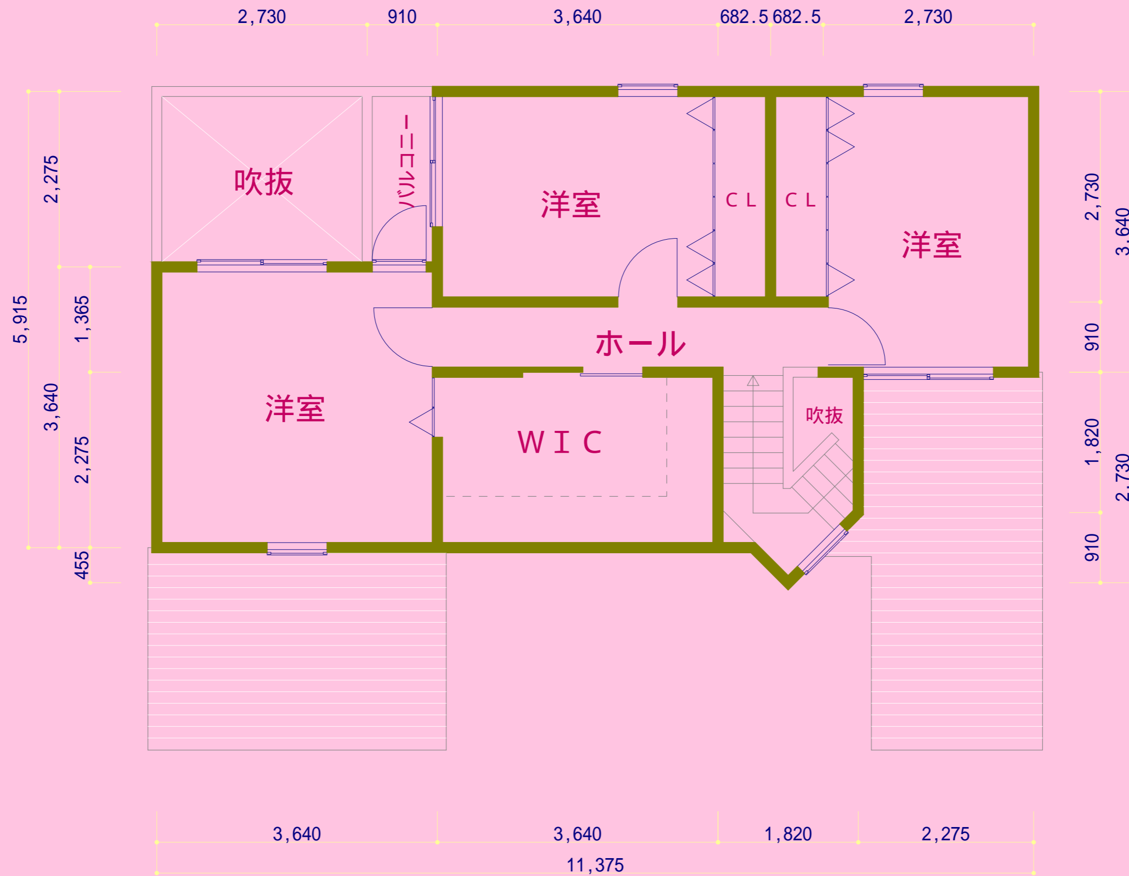
3階平面図
